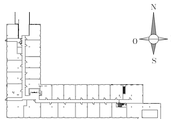
ÉTAGE 1 - RDC
